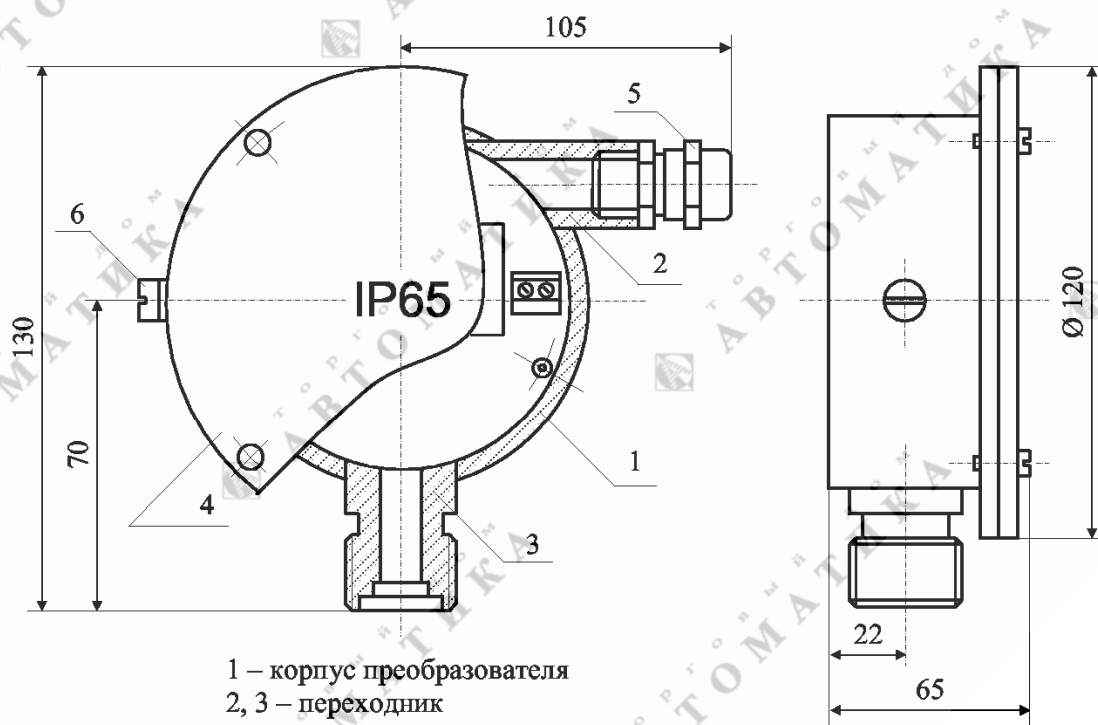
Рис. 2.1. Корпус ИП из алюминиевого сплава
