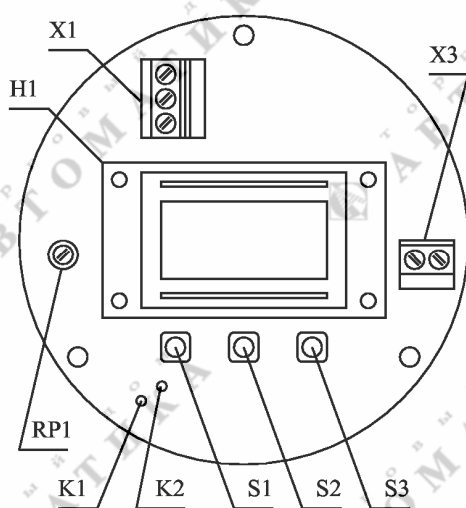
Рис. 1.2. ПП АЖК-3101М.х для корпуса из стали 12Х18Н10Т
