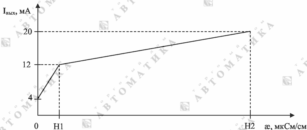
Рис. 3. Зависимость выходного тока от УЭП
