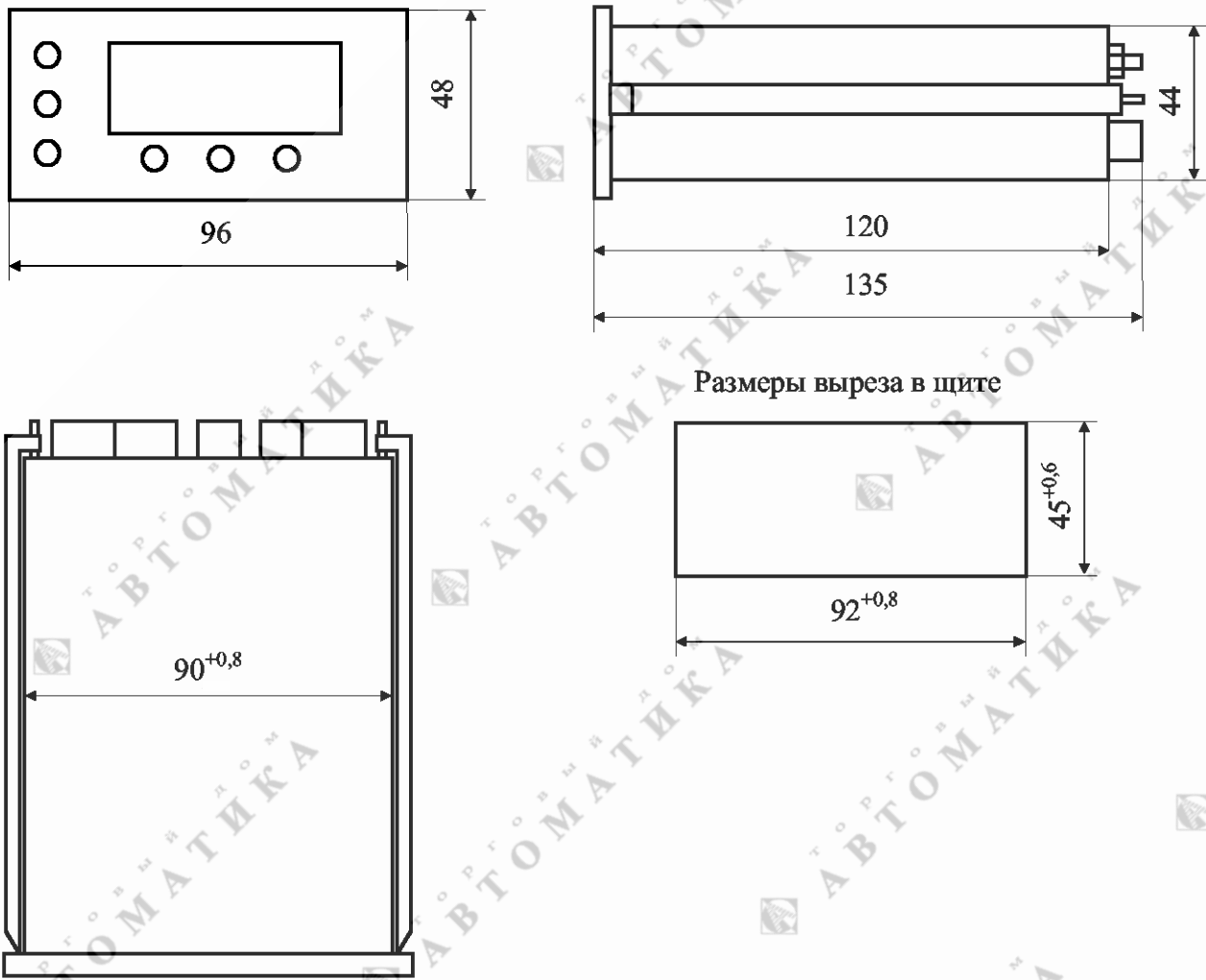
Рис. 3. Корпус измерительного прибора
