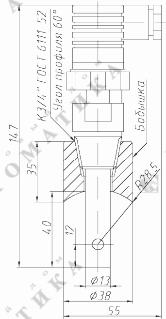
Рис. 1.4. ПП проточного типа высокотемпературный
