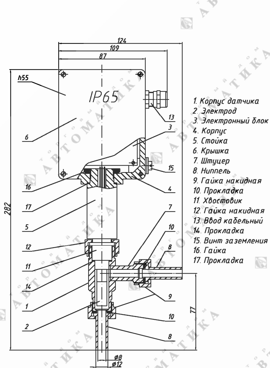
Рис. 1.1. ПП проточного типа с ниппелями под приварку
