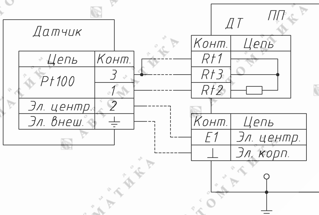
Рис. 2. Подключение высокотемпературного кондуктометрического датчика к первичному преобразователю прибора АЖК-3101М.Х.ВТ
