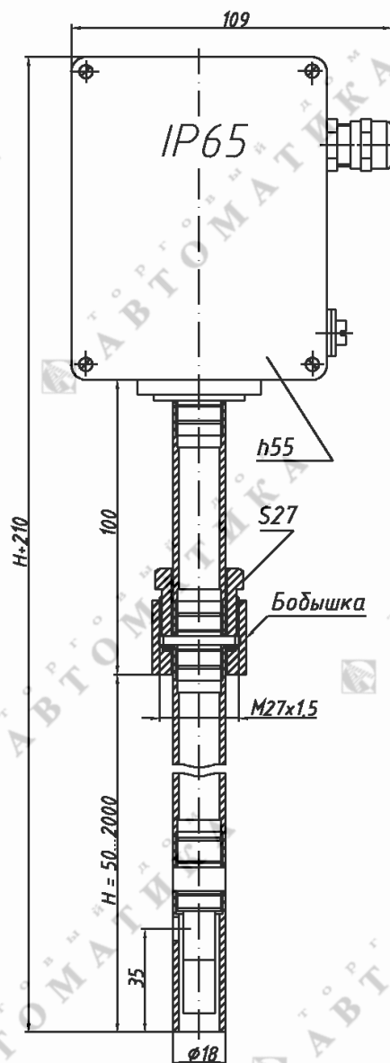
Рис. 1.2. ПП погружного типа
