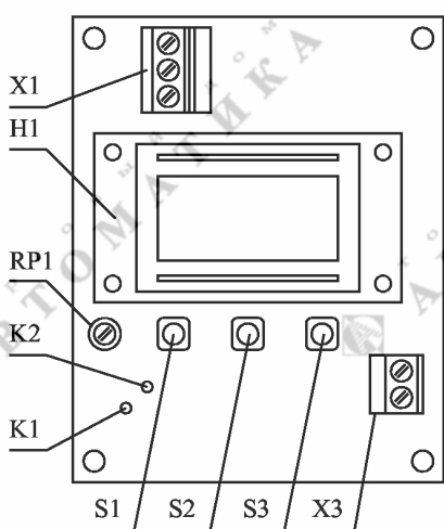
Рис. 1.1. ПП АЖК-3101М.х для корпуса из алюминиевого сплава
