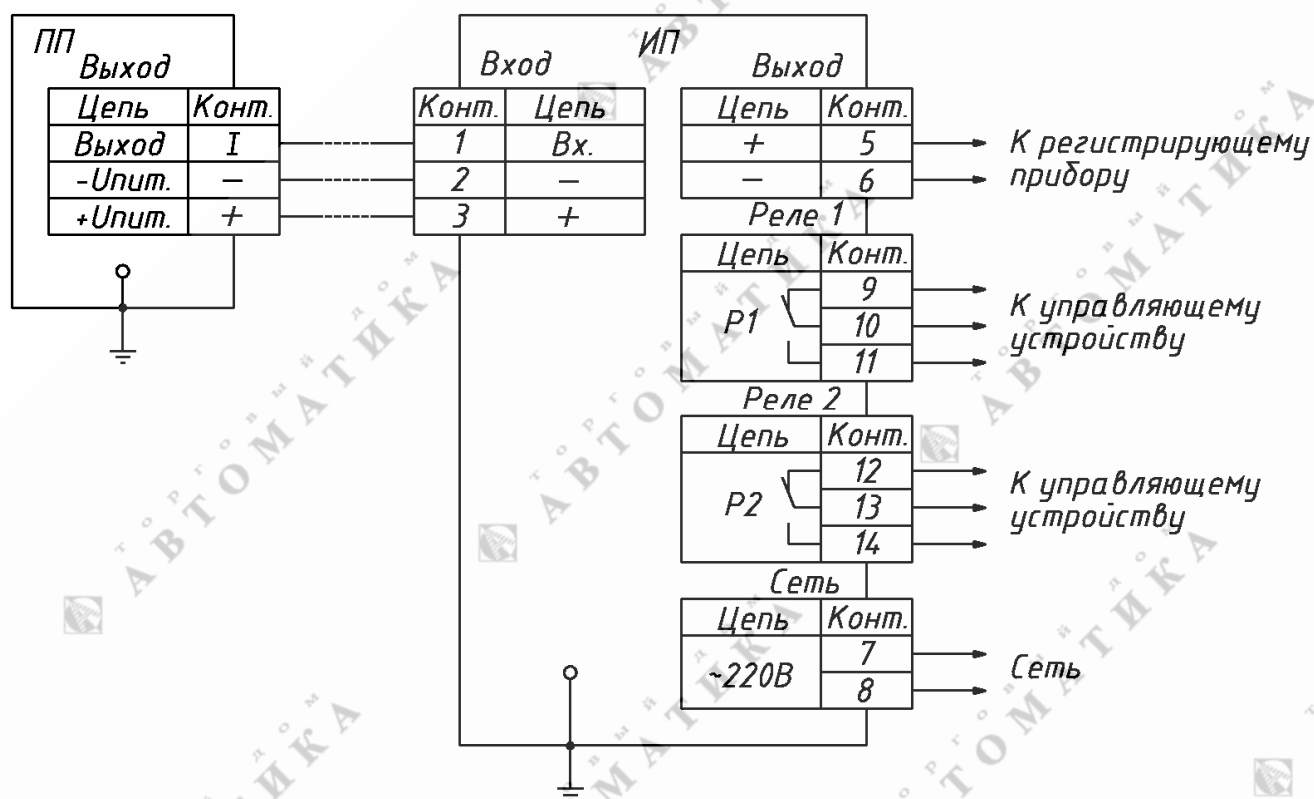
Рис. 1. Схема внешних соединений для АЖК-3101М.Х
