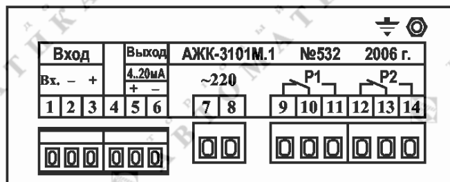
Рис. 2.2. Внешний вид задней панели
