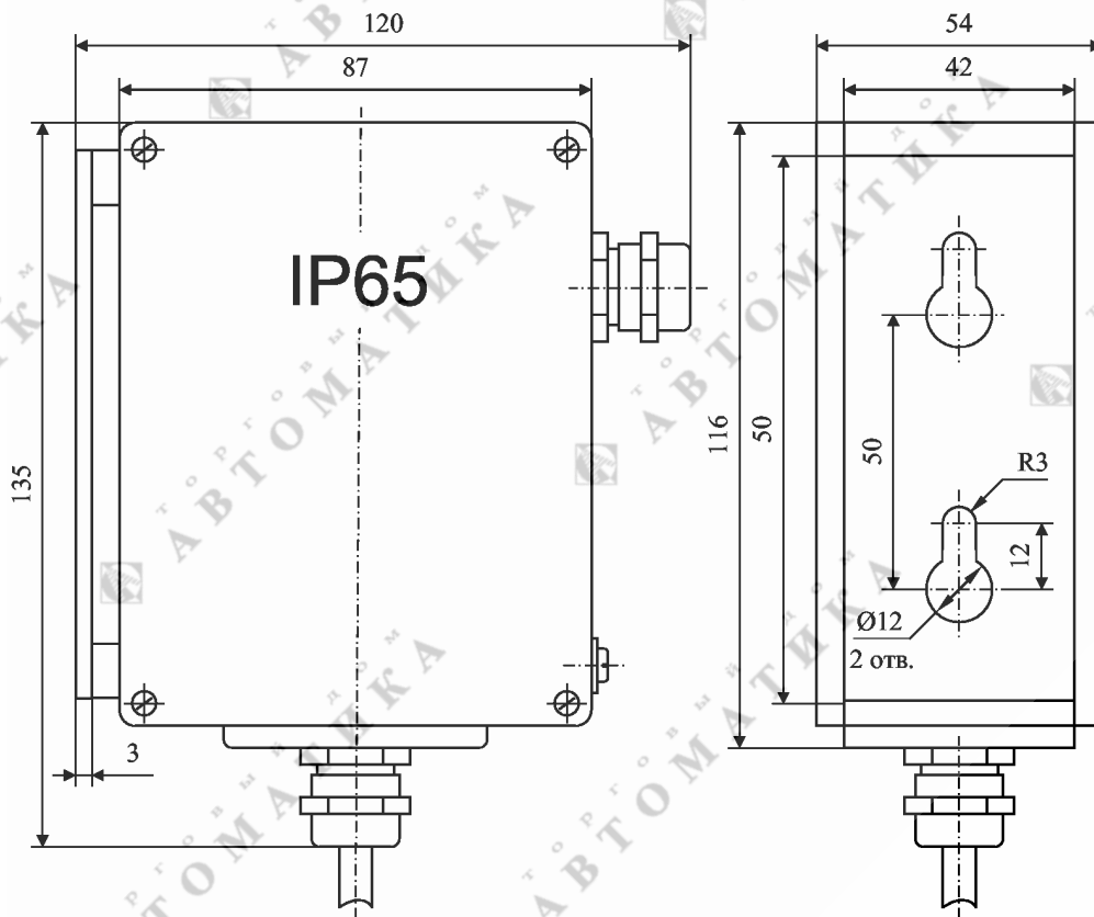
Рис. 2.4. Корпус ПП для навесного монтажа
