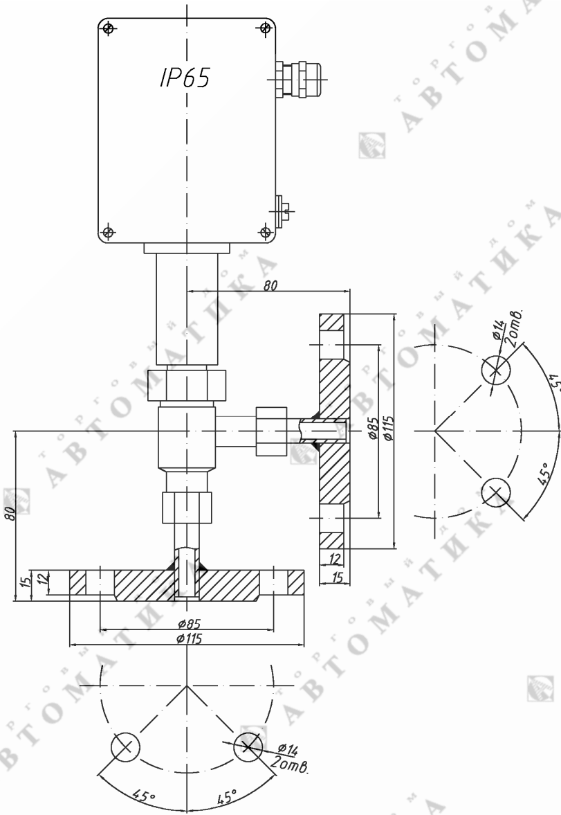
Рис. 1.3. ПП проточного типа с фланцами
