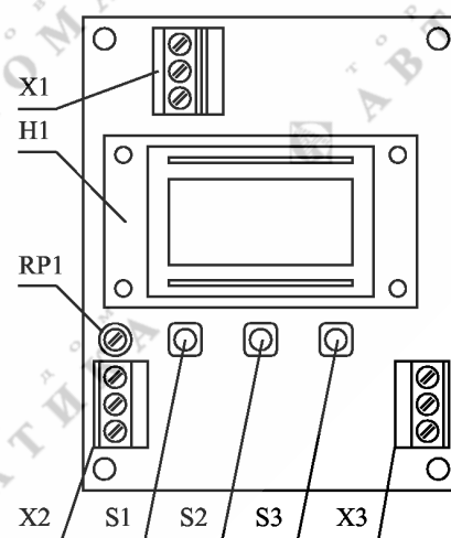
Рис.1.3. ПП АЖК-3101М.х.ВТ для корпуса из алюминиевого сплава
