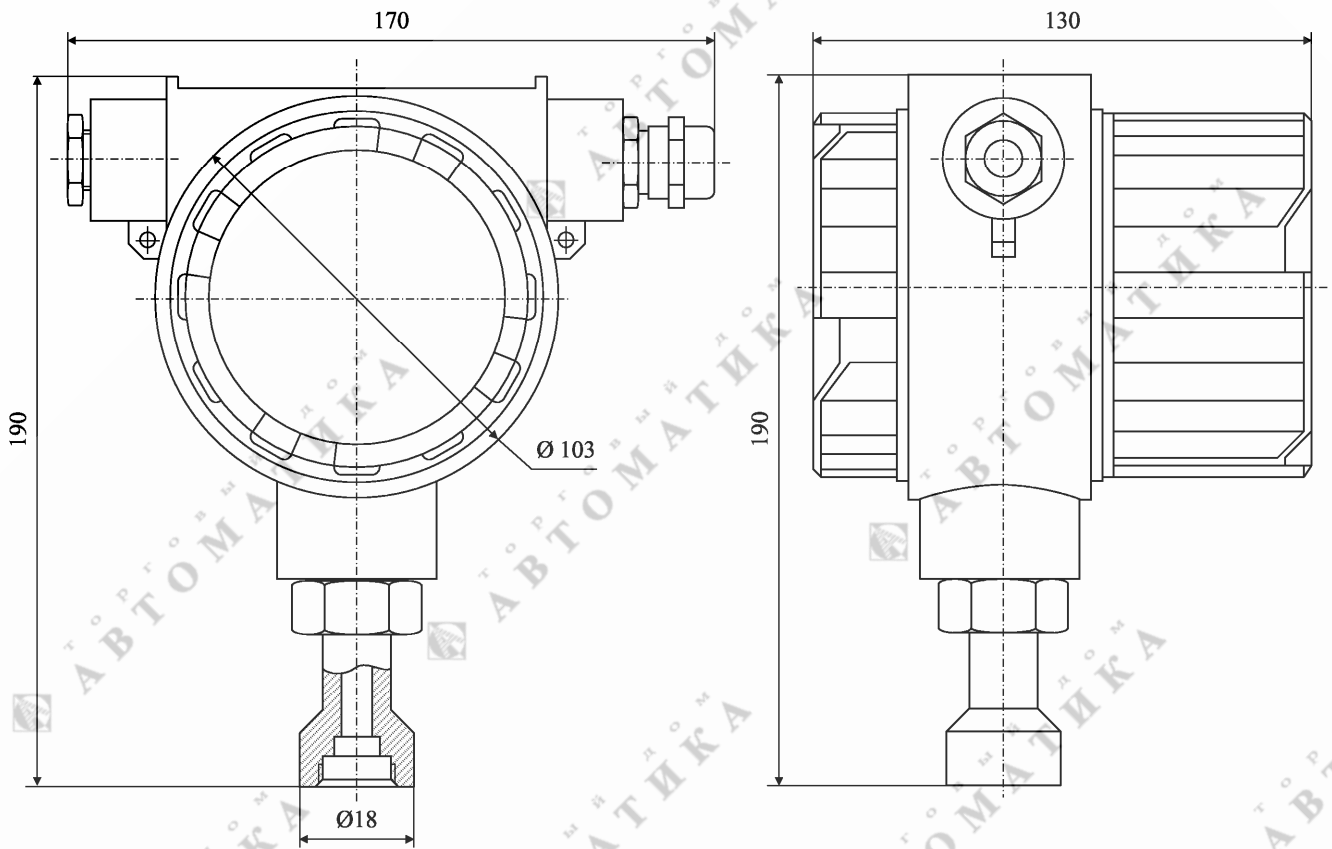
Рис. 2.3. Корпус ПП с индикацией
