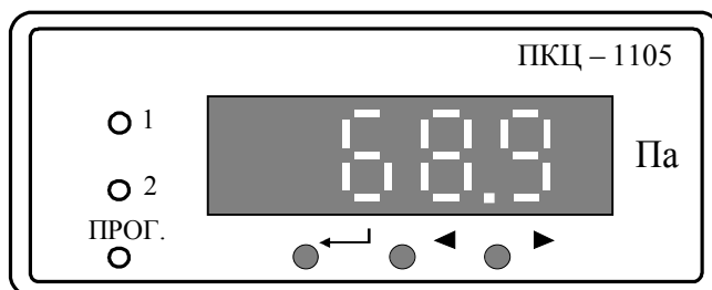
Рис. 1а. Внешний вид передней панели
