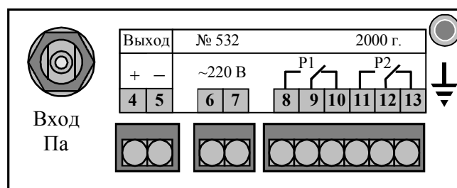
Рис. 1б. Внешний вид задней панели
