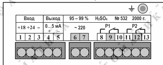
Рис. 2а. Внешний вид передней панели ИП
