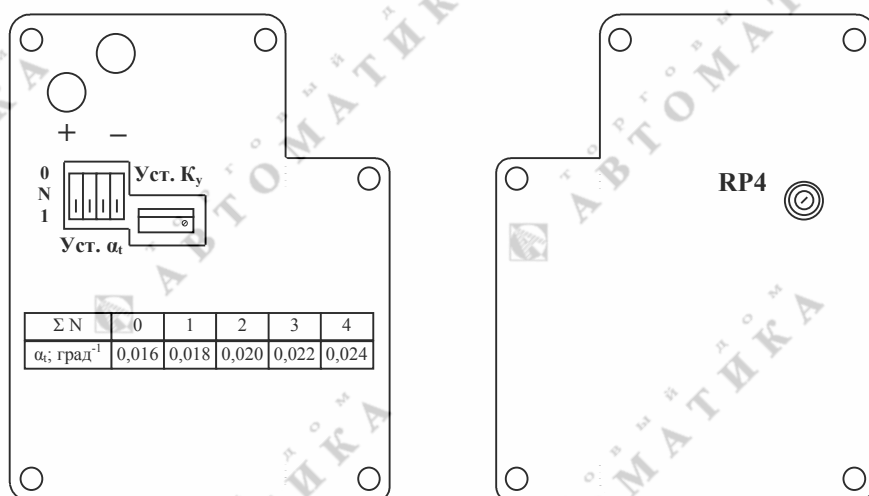
Рис. 1. Расположение органов регулировки ПП
